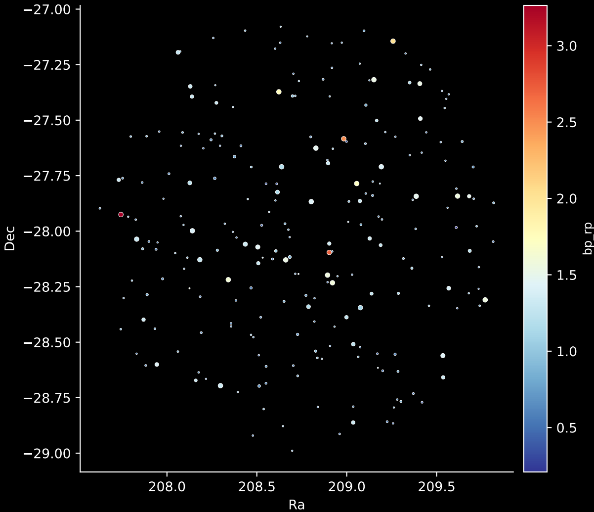
GALAH DR4 Field: [8340] Stars: 239
