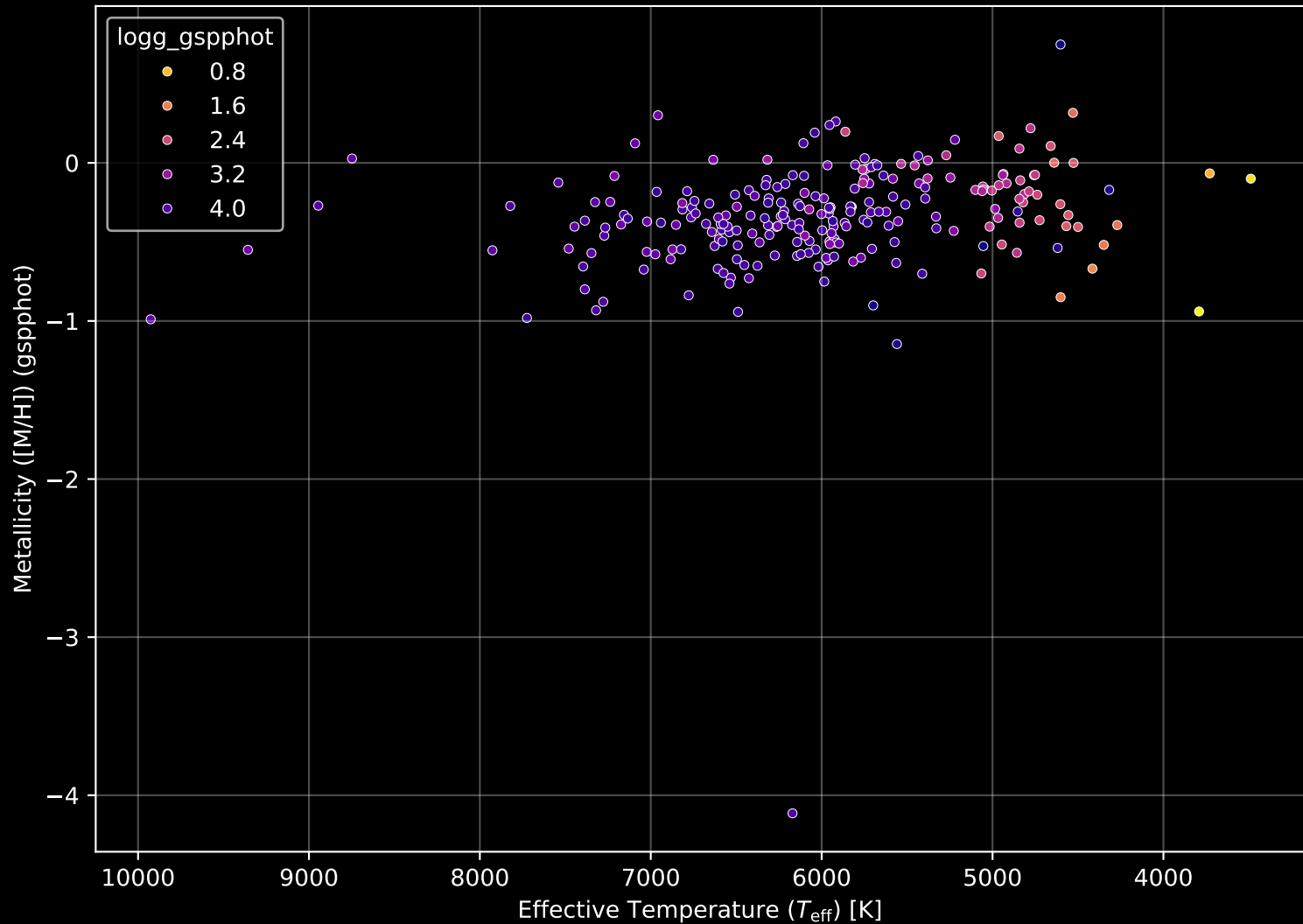
GALAH DR4 Field: [8340] Stellar Population Parameters (n= 239)
