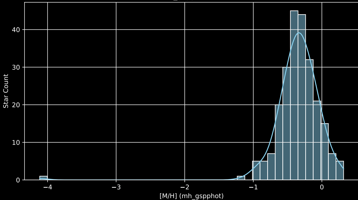
GALAH DR4 Field: [8340] [M/H] (mh_gspphot) (n= 238)
