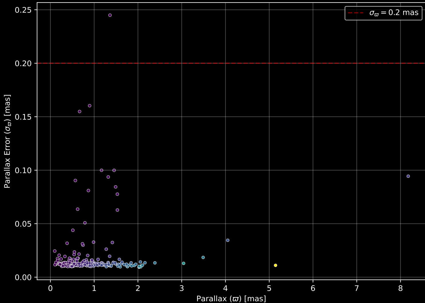
GALAH DR4 Field: [8340] Parallax Quality (n= 239)
